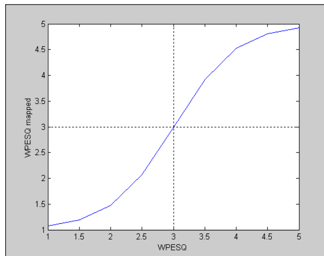
Fig. 1. The Barriac et al mapping function
