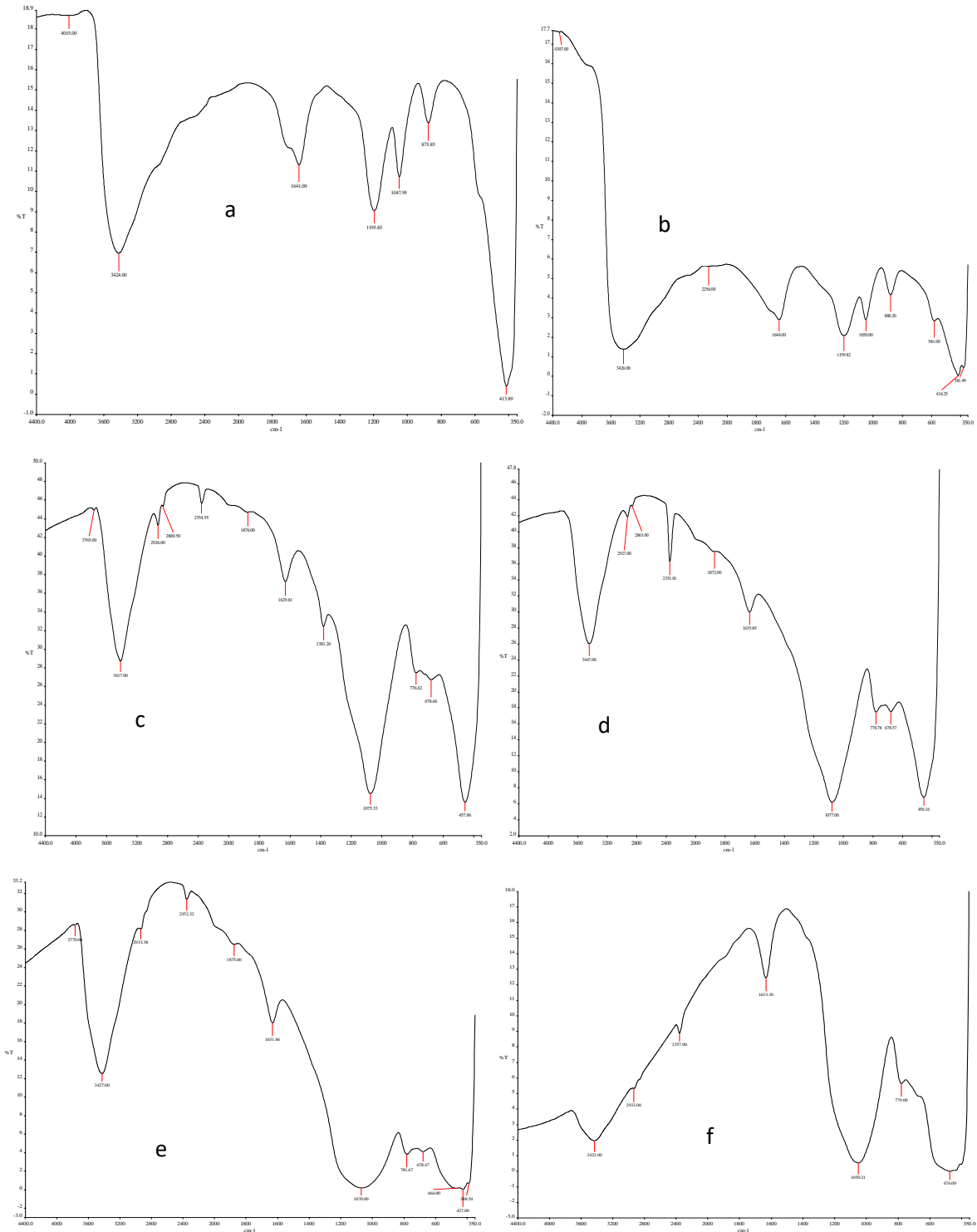
Fig. 5. The FTIR Spectrum of (a) JF (b) JA (c) JCI (d) JC2 (e) MN (f) CN
